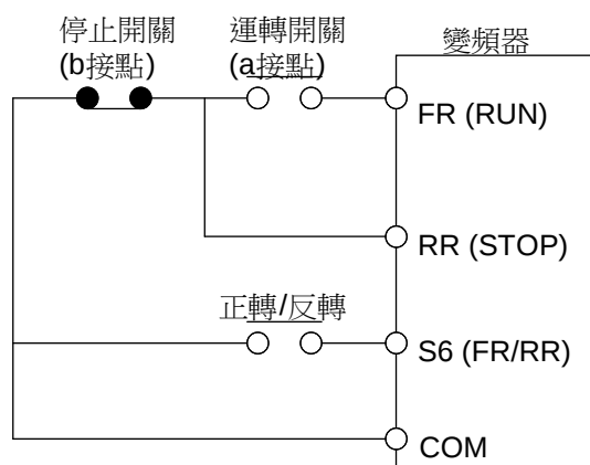
圖. 三線式運轉配線例
