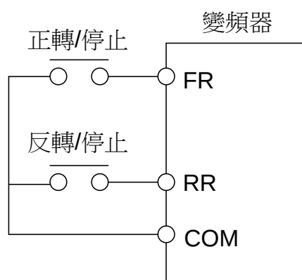
圖. 二線式運轉配線例
